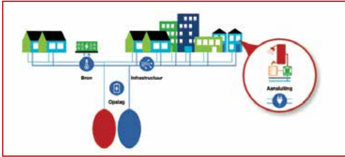
Figuur 1 Buurtwarmtenet zeer-lage-temperatuur: per huis warm je het water met een individuele waterwarmtepomp op naar de juiste temperatuur voor verwarming en warm tapwater
